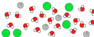
FIGURE 1.2 – L'eau de mer est un mélange constitué de molécules \text{H}_2\text{O} et d'ions \text{Na}^+ et \text{Cl}^- .
