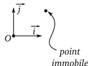
FIGURE 11.1 – Un objet sur lequel les forces se compensent peut rester immobile. Un objet immobile est soumis à des forces qui doivent se compenser.
