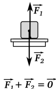
FIGURE 11.1 – Un objet sur lequel les forces se compensent peut rester immobile. Un objet immobile est soumis à des forces qui doivent se compenser.
