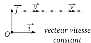
FIGURE 11.2 – Un objet sur lequel les forces se compensent peut avoir un mouvement rectiligne et uniforme. Un objet en mouvement rectiligne et uniforme est soumis à des forces qui doivent se compenser.
