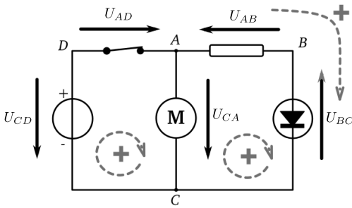
FIGURE 16.5 – La loi des mailles signifie que la somme des différences de potentiels dans une maille est nulle.
