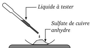
FIGURE 1.3 – La présence d'eau est confirmée par la coloration en bleu du sulfate de cuivre anhydre
