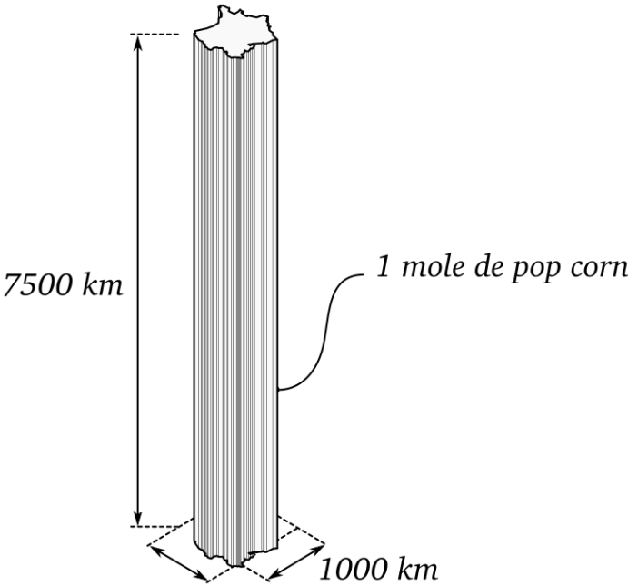
FIGURE 5.1 – Une mole de pop-corn couvrirait la France sur 7500 km de haut.
