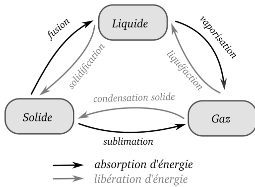
FIGURE 6.1 – Noms des différents types de changements d'états.
