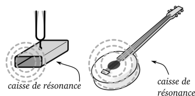
FIGURE 12.2 – Le son du diapason est amplifié grâce à une caisse de résonance. La corde métallique d'un instrument de musique est fixée sur une caisse en bois pour que le son émis soit plus fort.
