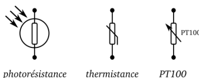
FIGURE 16.8 – Symboles électriques de différents capteurs résistifs.
