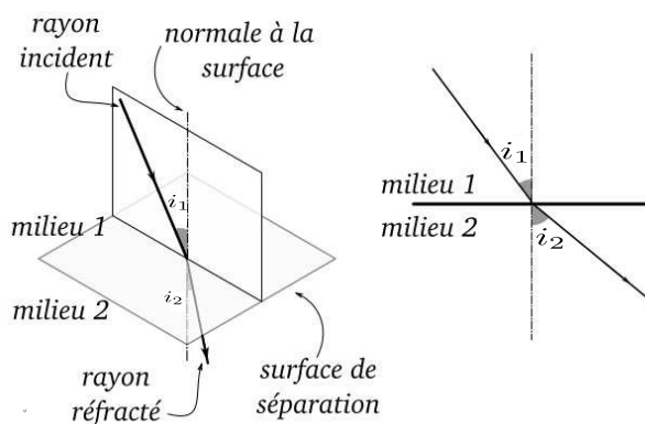
FIGURE 14.2 – La réfraction est le changement de direction de propagation d'un rayon lumineux quand il change de milieu. Les angles d'incidence i_1 et de réfraction i_2 sont liés aux indices optiques n_1 et n_2 des deux milieux grâce à la loi de Snell-Descartes.
