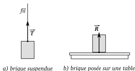
FIGURE 10.4 – Les interactions de contact nécessitent que les objets interagissants se touchent. Le système étudié est la brique.
