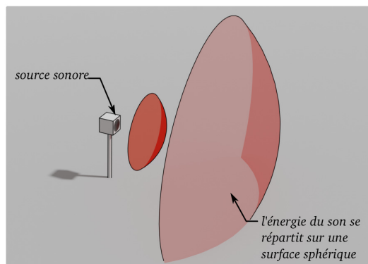
FIGURE 12.7 – La puissance transportée par une onde sonore (une énergie par seconde) se répartit sur une surface de plus en plus grande en s'éloignant de la source. L'intensité du son décroît.
