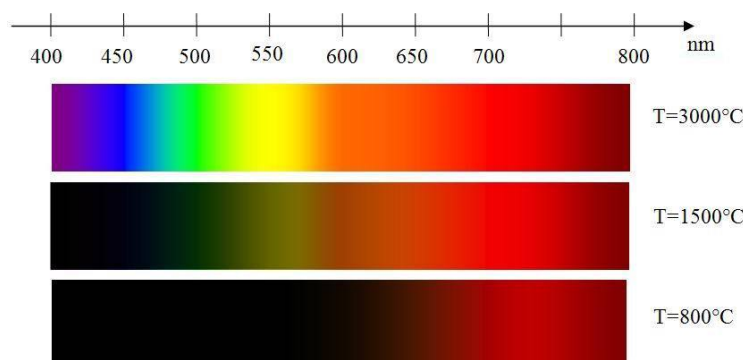
FIGURE 13.6 – Les spectres d'émission dépendent de la température du corps émetteur.
