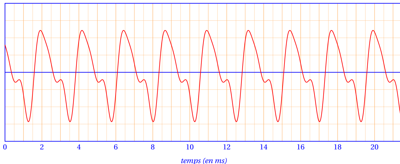
FIGURE 12.4 – Note d'un instrument de musique. On observe la présence d'un motif périodique.
