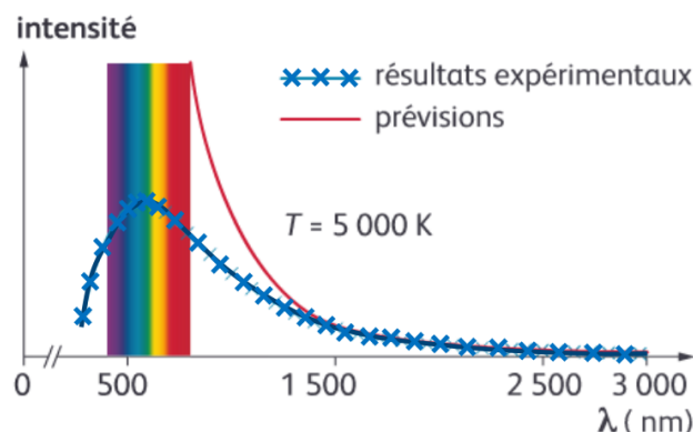
Figure 2: Évolution de l'intensité lumineuse émise par un corps chaud en fonction de la longueur d'onde.
